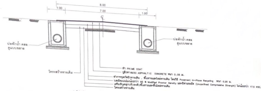
รูปตัดโครงสร้างทาง (A - A) NOT TO SCALE ช่วงที่ 1
