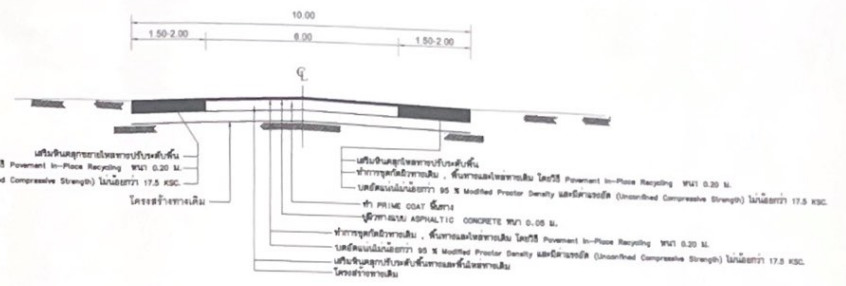
รูปตัดโครงสร้างทาง (C - C) NOT TO SCALE ช่วงที่ 3
