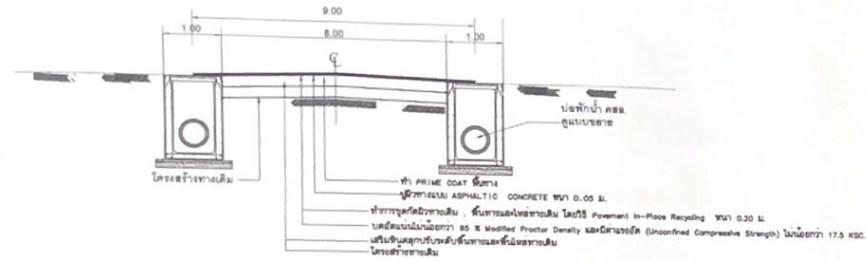
รูปตัดโครงสร้างทาง (B - B) NOT TO SCALE ช่วงที่ 2
